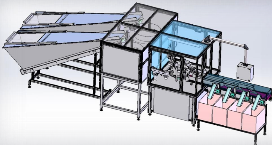
Rundtakt-Montage-Maschine zur Rasierschaum-Kappen-Montage
